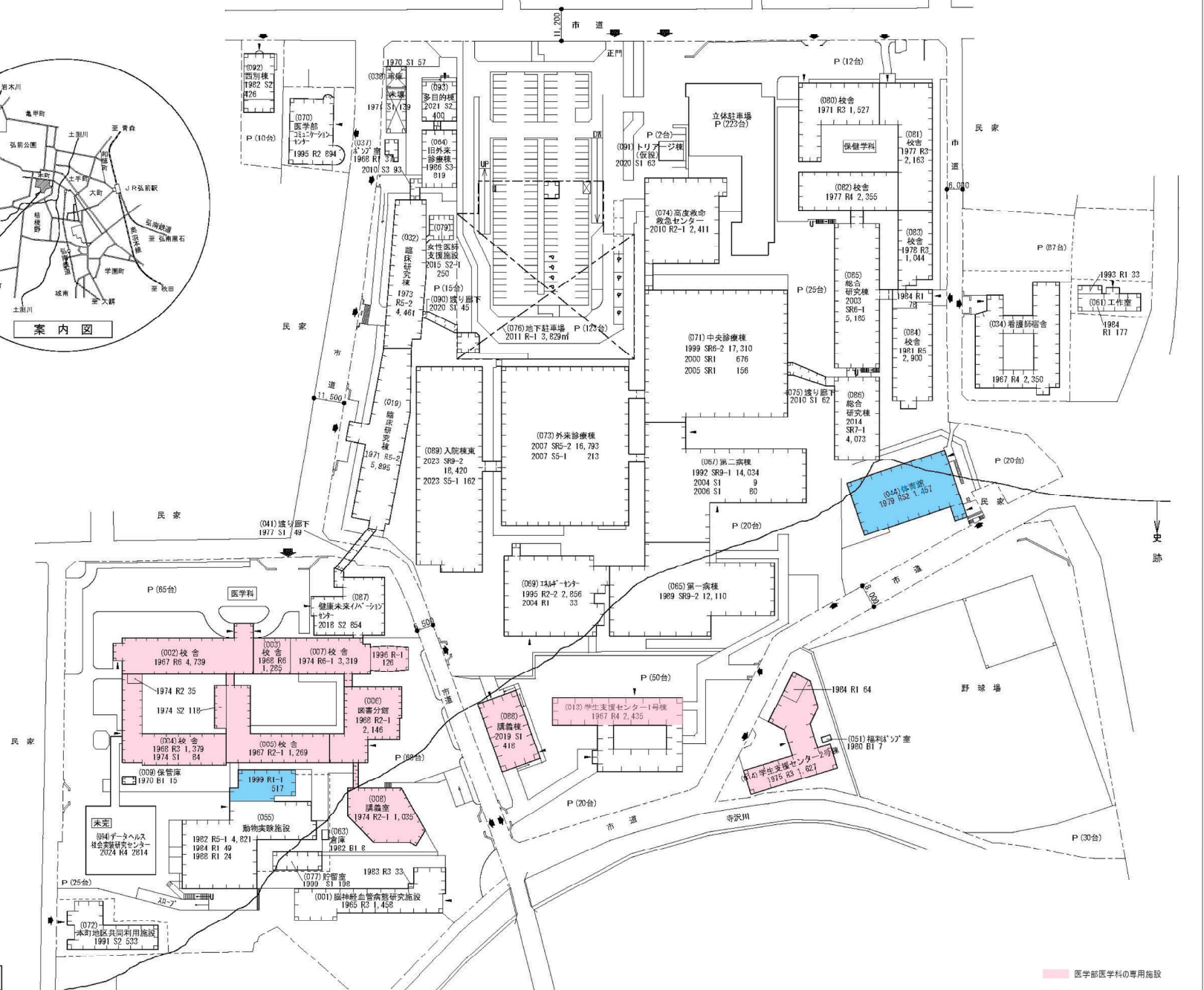
本町団地配置図S:1/1,500
